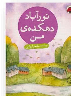
نورآباد دهکده من
